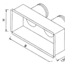
Plenum CS5 : cf. p.160
