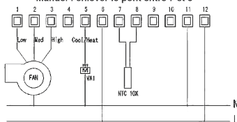
Câblage :
