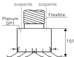
KD monté avec Plenum DP1
