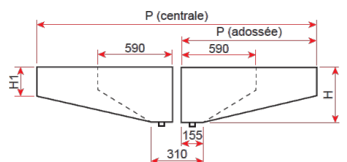
Hotte Statique T
