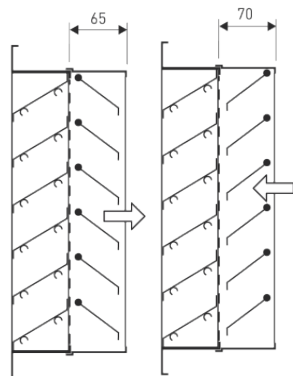
Clapet anti-retour monté (aspiration ou rejet)
