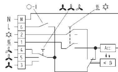
Câblage
