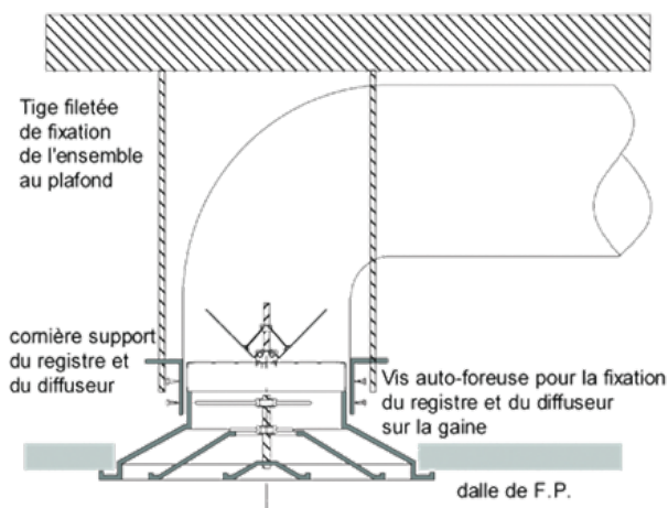
Diffuseur KRA sur dalle de faux plafond
