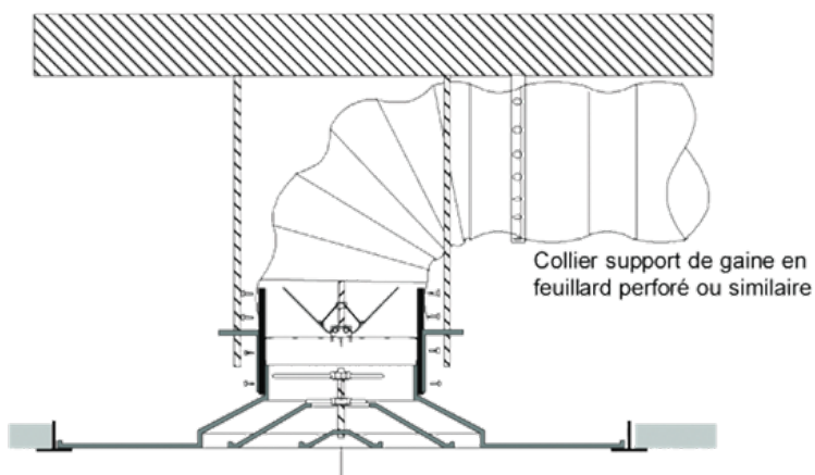
Diffuseur KRAFP sur élément porteur de faux plafond
