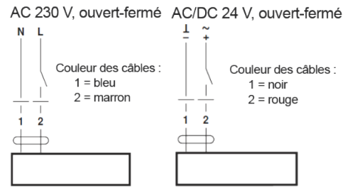
Câblage LF230
