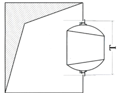
Dimension du trou sur gaine rectangulaire
