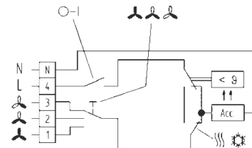
Câblage
